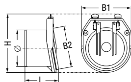
A ilustração mostra Ø 250 - Ø 638
