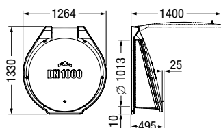
A ilustração mostra Ø 1000
